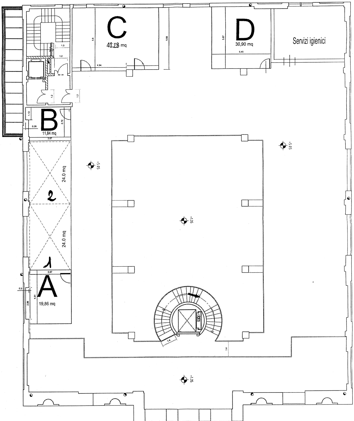
PIANTA PIANO MEZZANINO Scala 1:100
