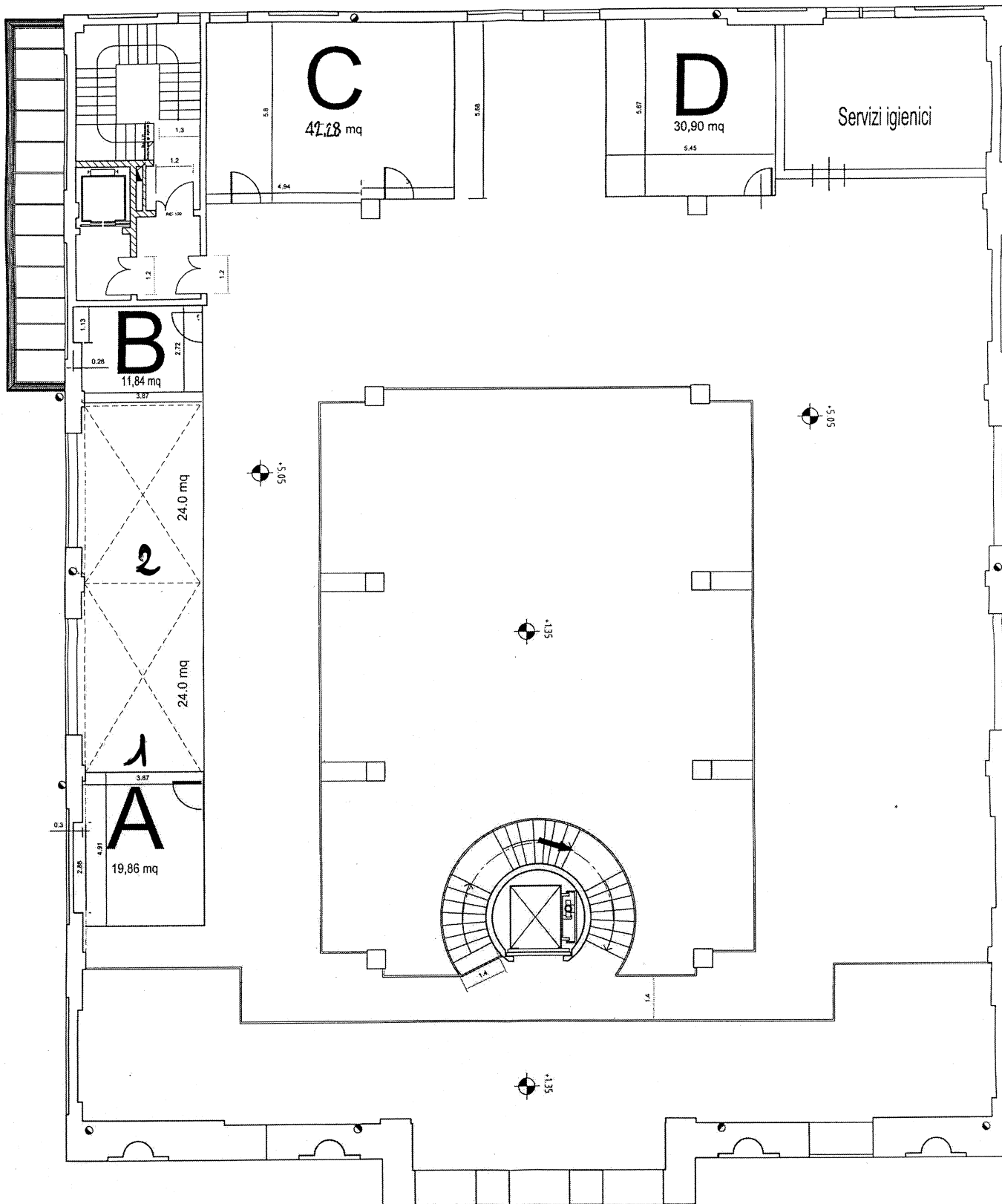
PIANTA PIANO MEZZANINO Scala 1:100
