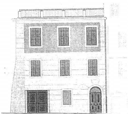
PROSPETTO OVEST SU VIA MARIANI
